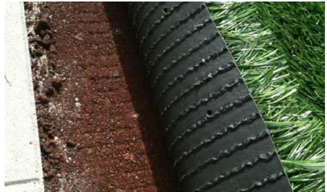
Die Vulkanerde wird eingebaut (links), danach wird darüber der Kunstrasen verlegt (rechts)
